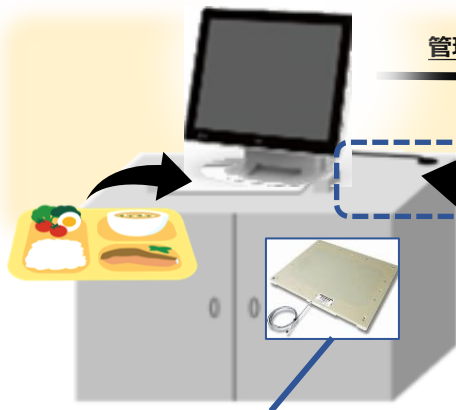
アンテナ (タグ読み取り用) TR3-WA103 550(W)×450(D)×17(H)mm 約1.7kg
